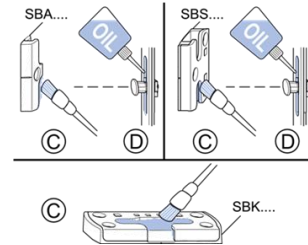
Punkty smarowania
