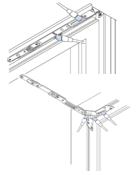
Rozwórka ( widok z dołu )
