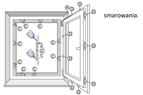
Punkty smarowania
