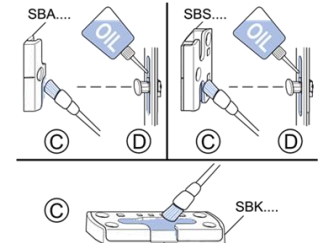
Punkty smarowania
