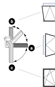
Test prawidłowego funkcjonowania okucia w oknie uchylno-rozwieranym
